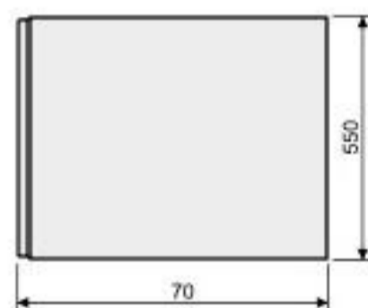
OWP/CLa rövid oldallap
